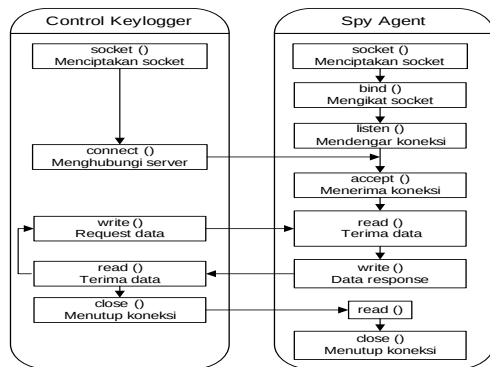
Gambar 4 : Mekanisme kerja control keylogger dan spy agent
