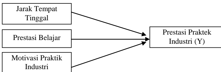
Gambar 1 Kerangka Penelitian
