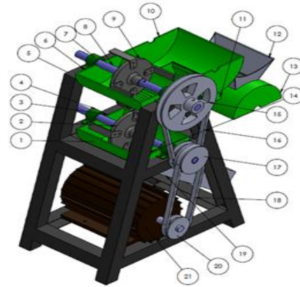
Gambar 2. Desain mesin perajang tembakau
